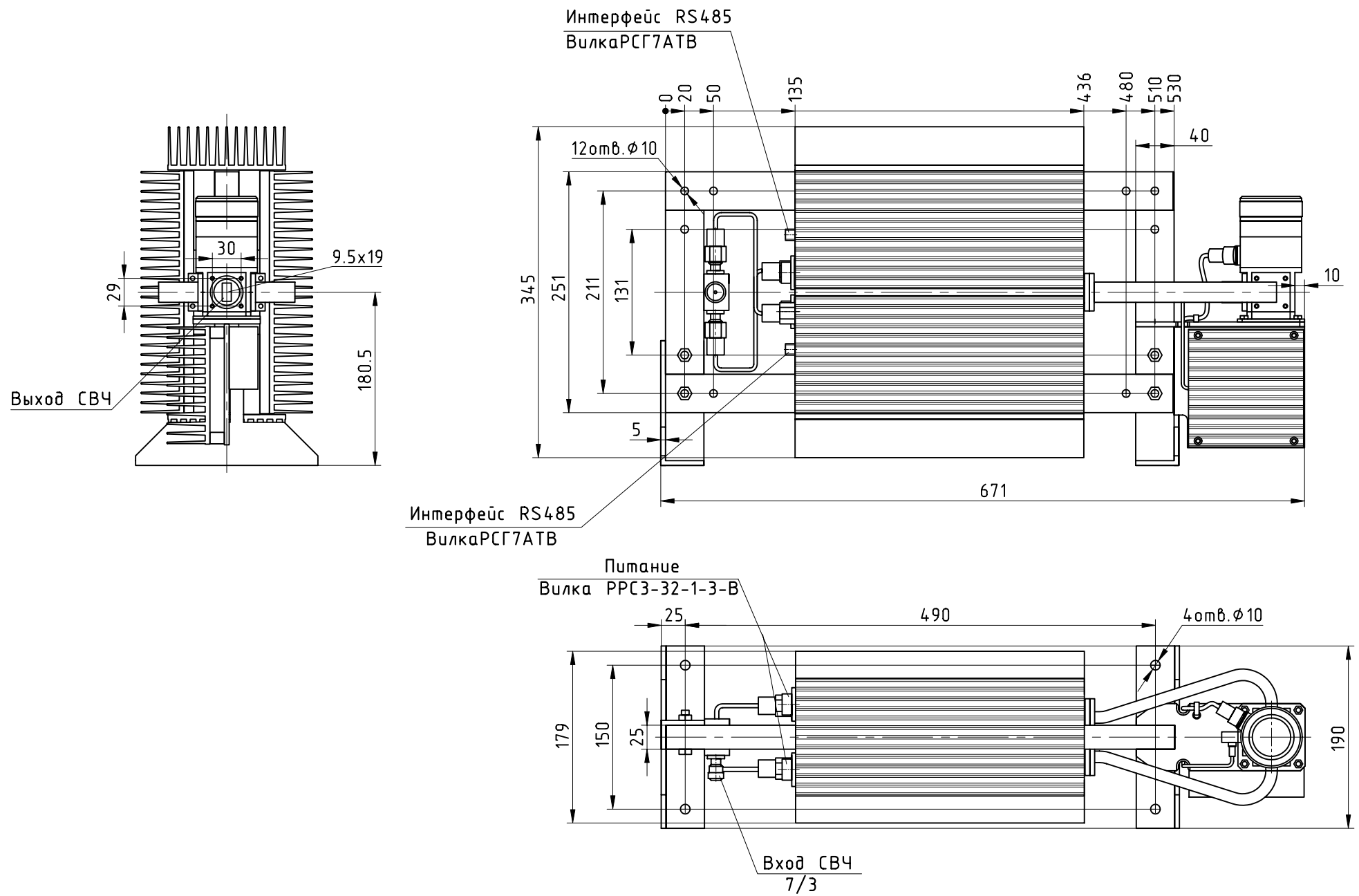
Блок резервированного усилителя мощности Ku-диапазона УМ1414-25Р (УМ1314-25Р)
